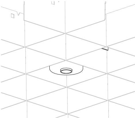
3D bottom view PUNTEO-N 1x1 S01 in Quadra 50H30
