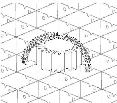
Top view PUNTEO-N 1x1 S01 in Quadra 30H30
